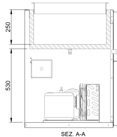
SEZ. A-A
